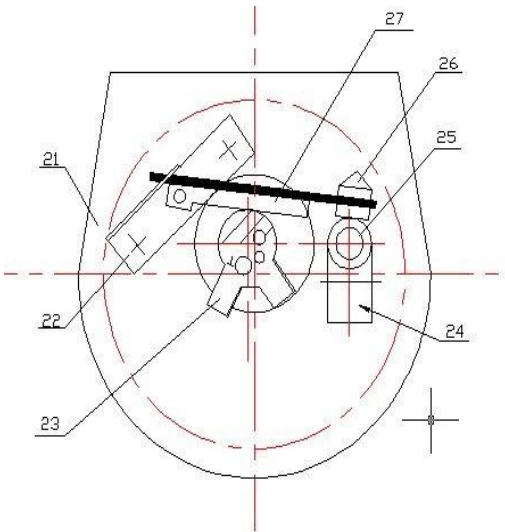
图 (二) 自吸进油
