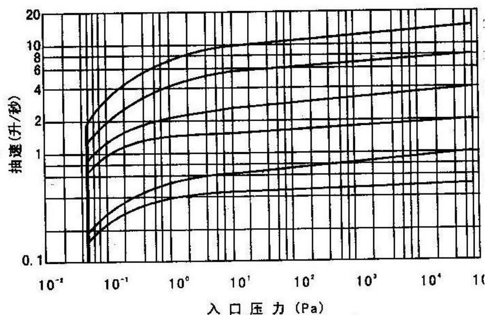
抽速特性曲线图 图(五)
