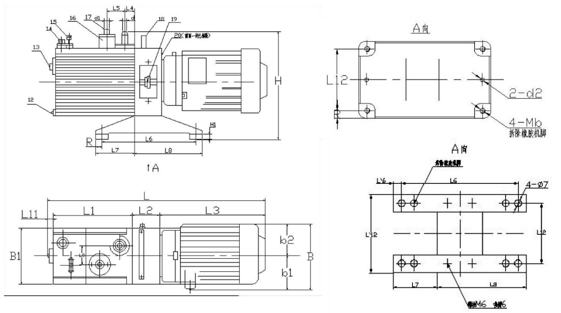
外形尺寸安装图（矩形管）
